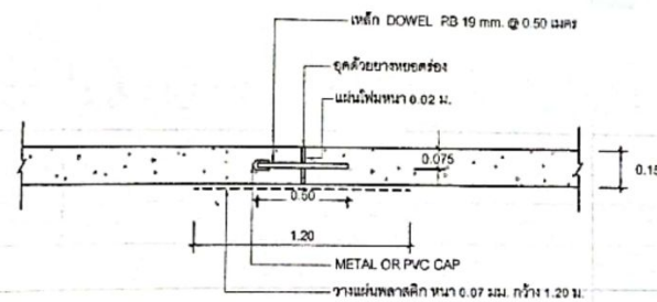
ขยาย EXPANSION JOINT SCALE 1:20
