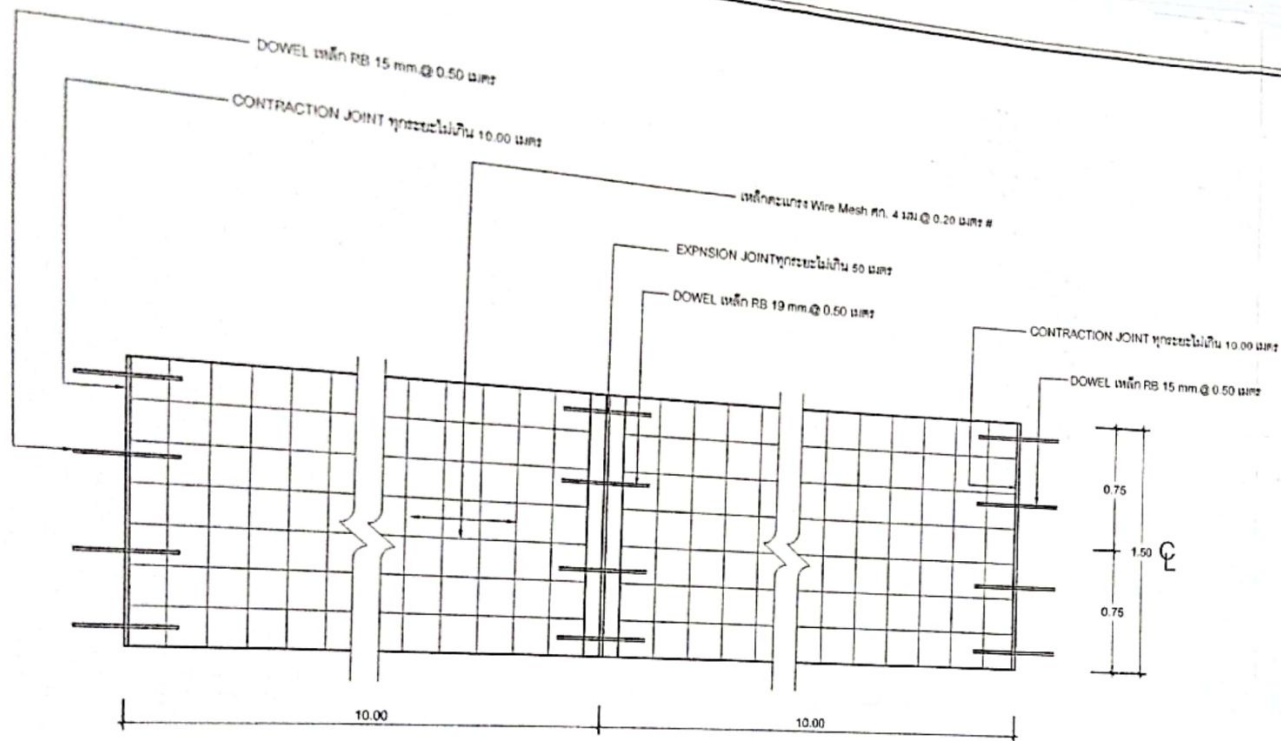
แปลนการวางเหล็กตะแกรง SCALE 1:20
