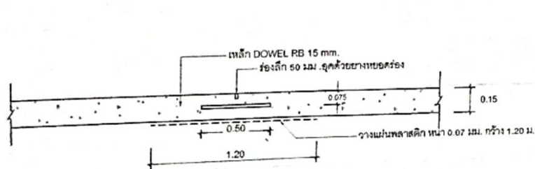
ขยาย CONTRACTION JOINT SCALE 1:20
