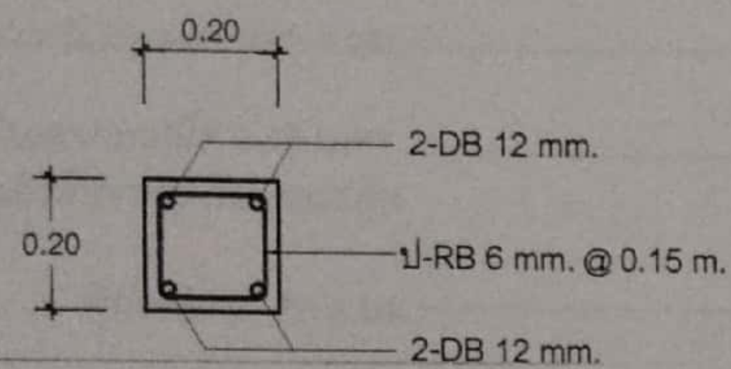
C1. ตอม่อ-หัวเสา
