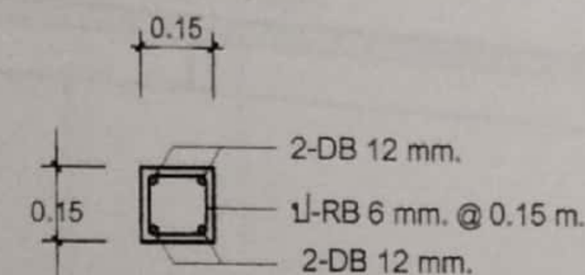
C2. ตอม่อ-หัวเสา
